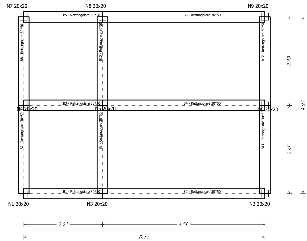
Pianta carpenteria coperture quota gronda-colmo
