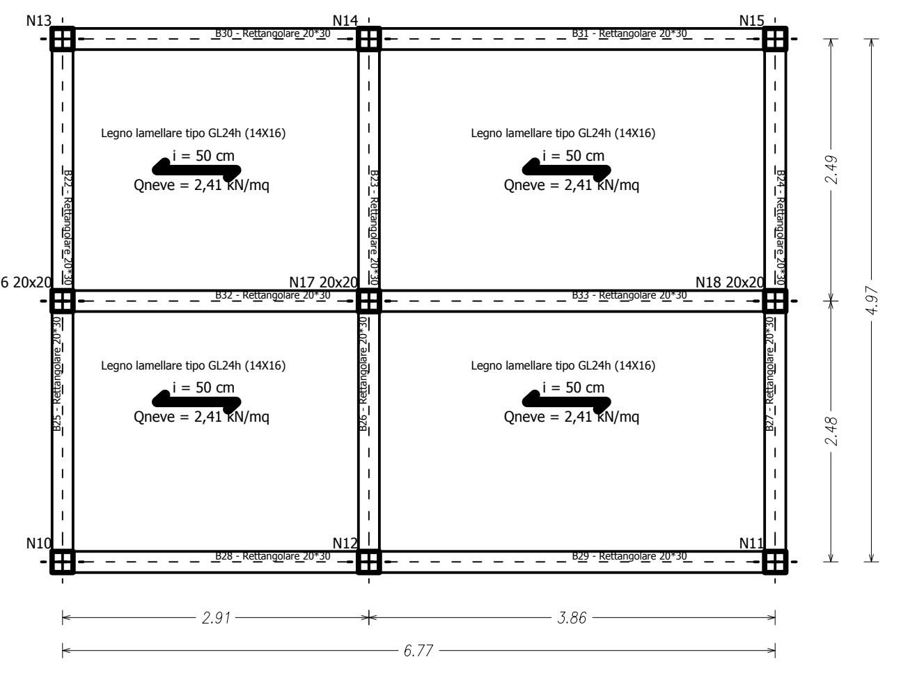
Pianta carpenteria coperture (quota linea di gronda)
