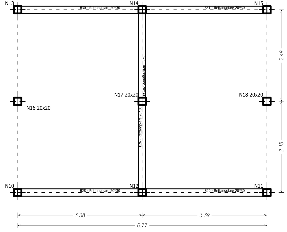
Pianta carpenteria coperture (quota linea di gronda)
