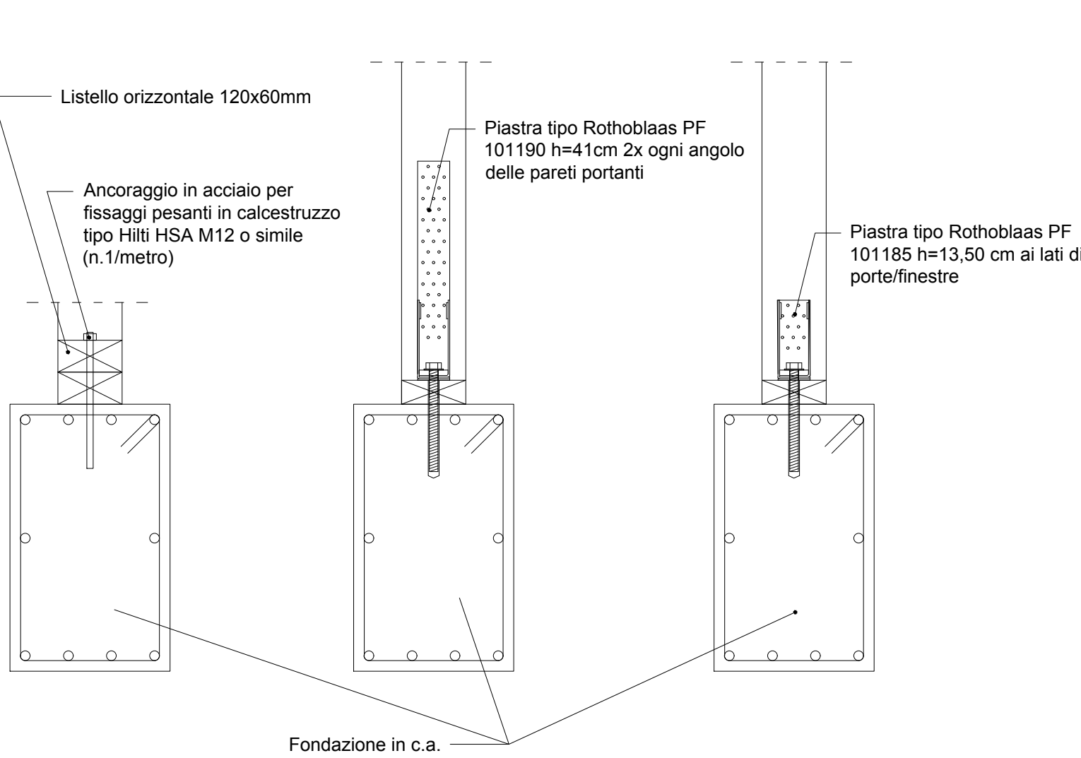
PARTICOLARI ANCORAGGI - Scala 1:10
