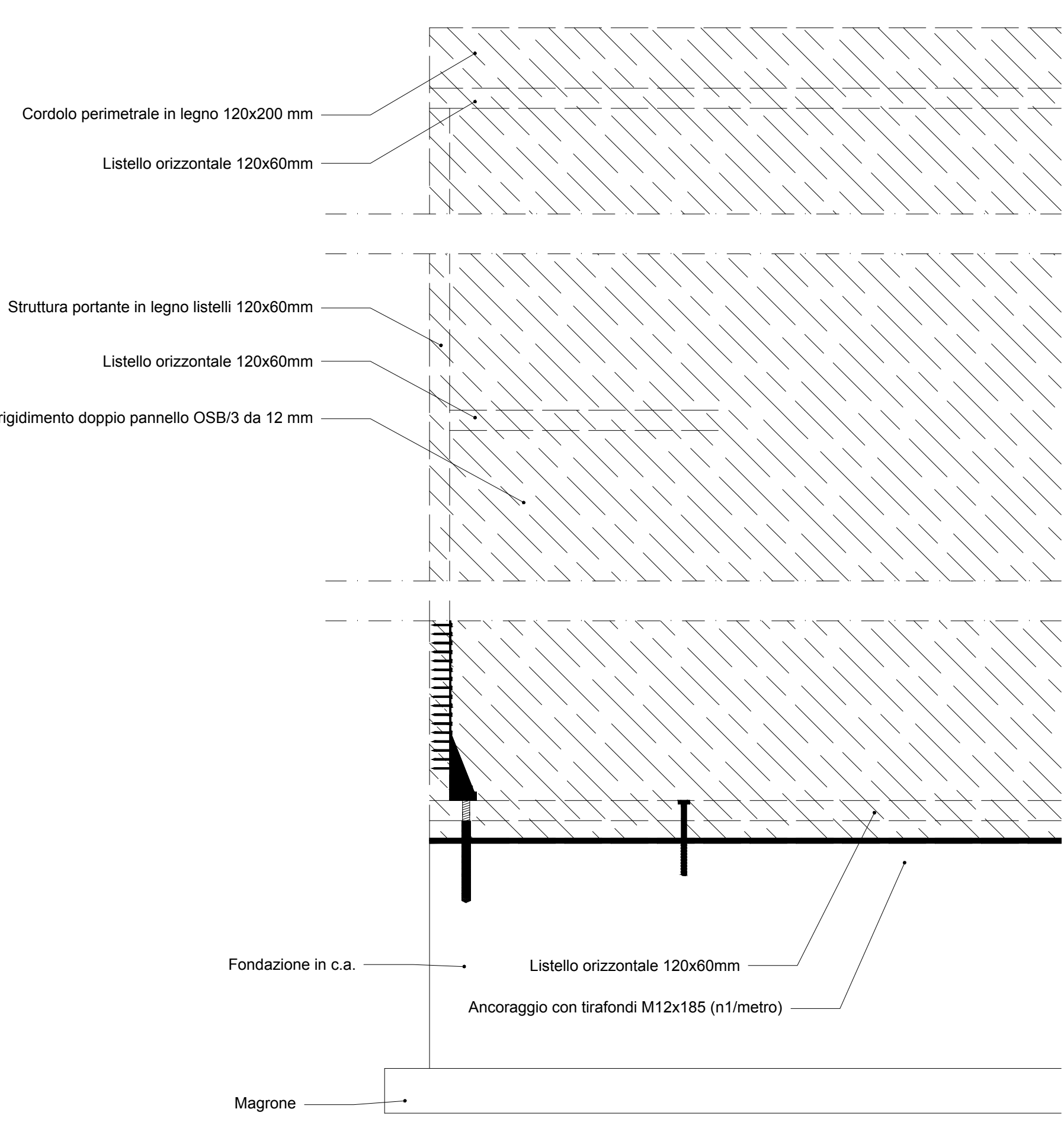
SCHEMA DEL TELAIO PORTANTE - Scala 1:10
