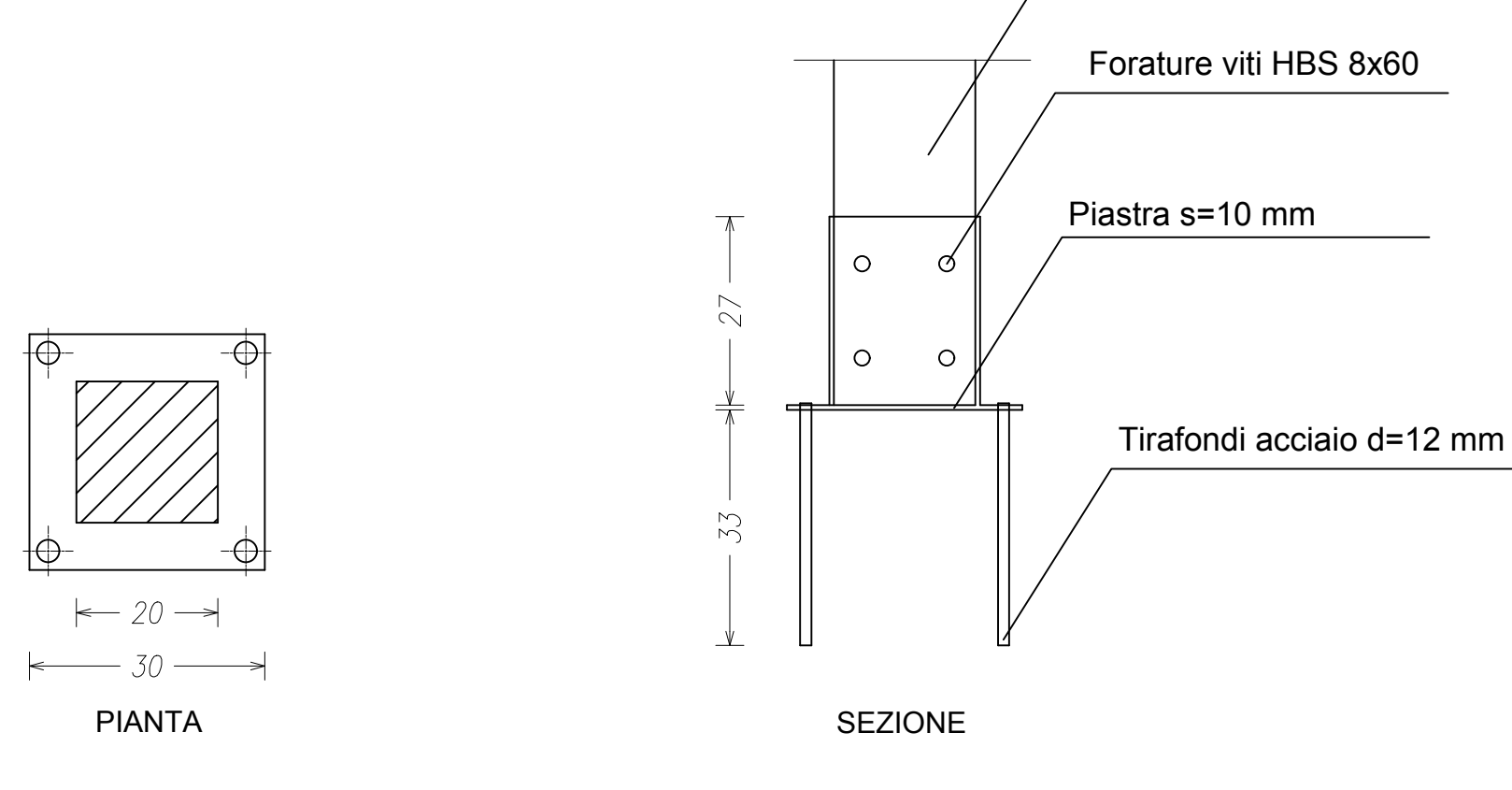
PARTICOLARI ESECUTIVI SCARPE - Scala 1:10
