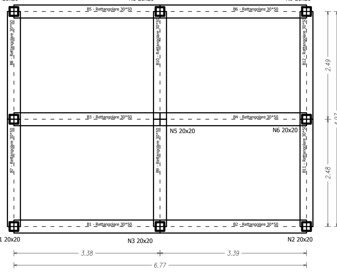
Pianta carpenteria delle fondazioni (0,00)
