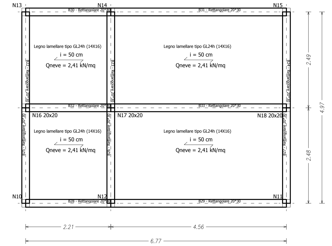
Pianta carpenteria coperture quota gronda-colmo
