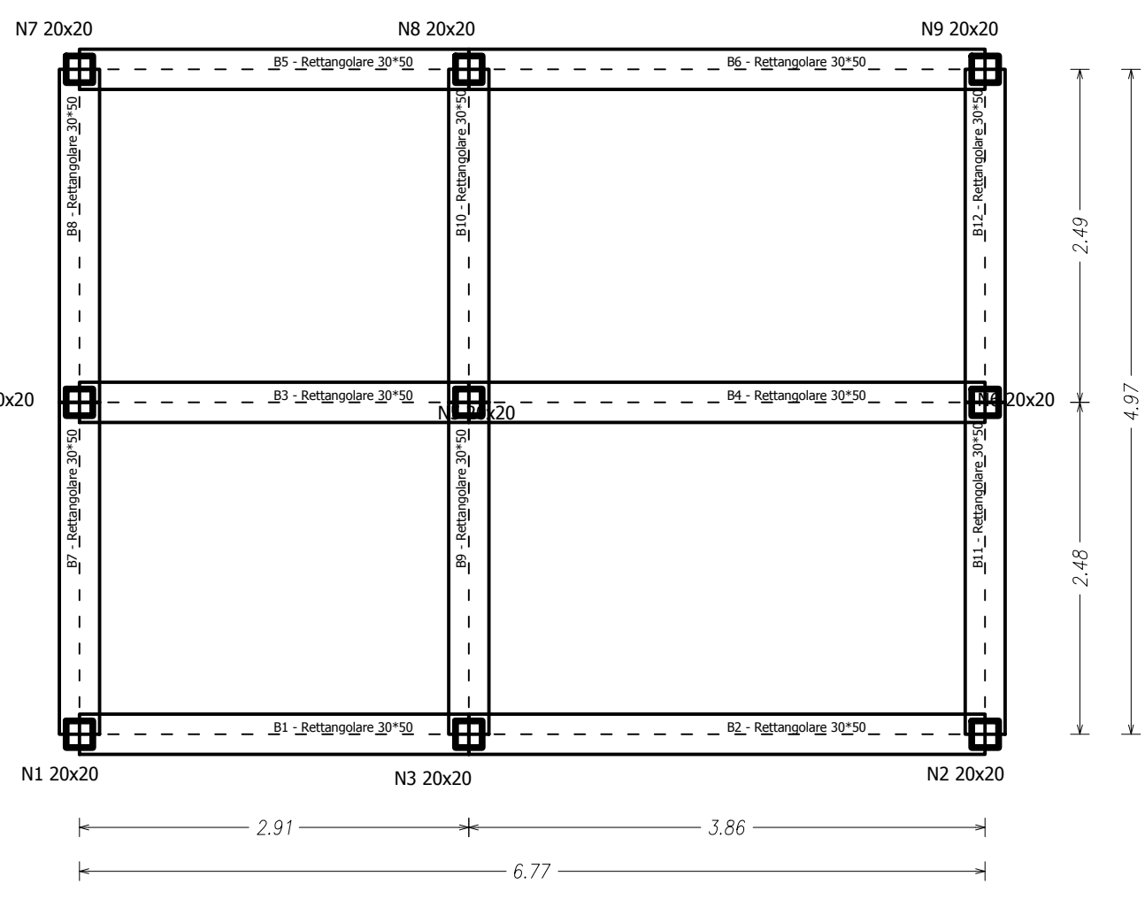
Pianta carpenteria delle fondazioni (0,00)
